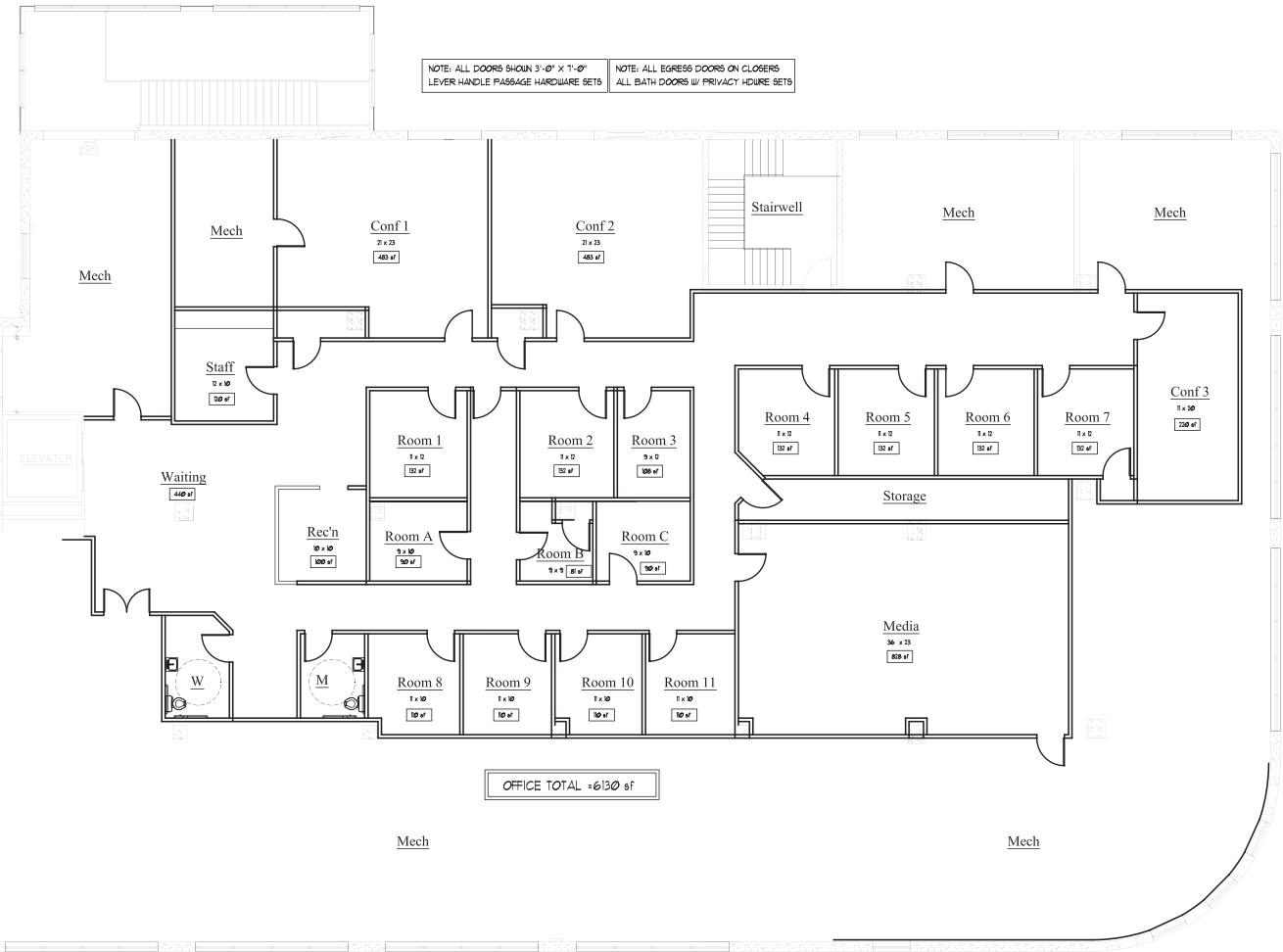
2 A-1 Lower Level Plan SCALE: 1/8" = 1'-0"
