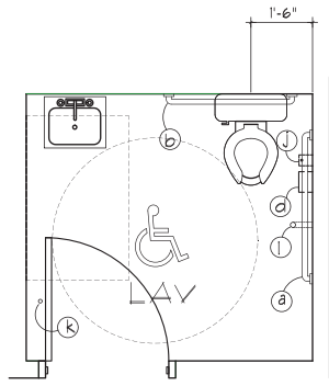
2 A-1 Typ. Bathroom Plan SCALE: 1/8" = 1'-0"
